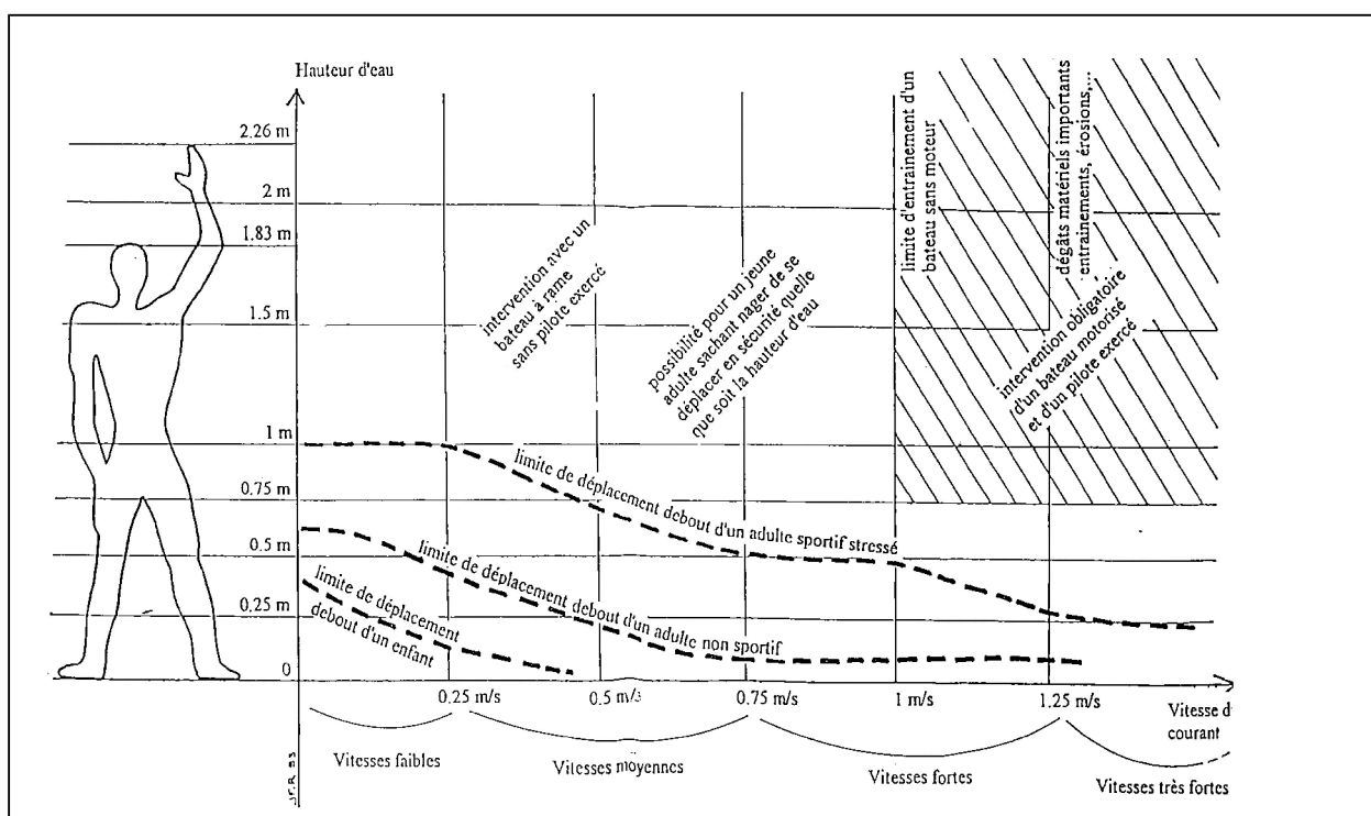
Figure 3 : Capacités de déplacement en fonction des hauteurs d'eau et des vitesses d'écoulement
