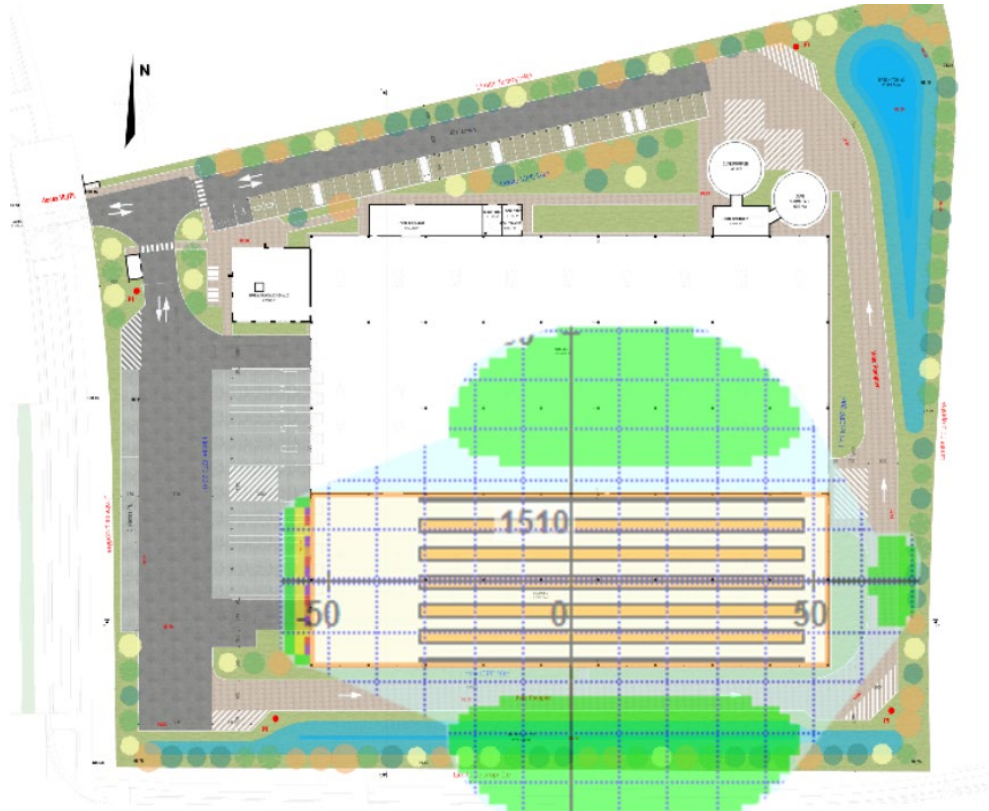
Zones d'effets thermiques : palette type 1510 - Cellule 2 Stockage 11,7 m
