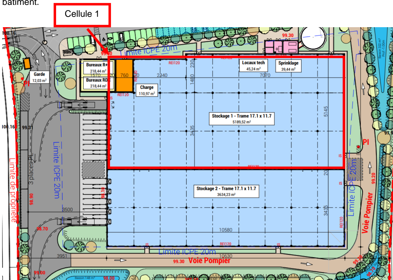
Figure 4: Découpage en cellule du site
