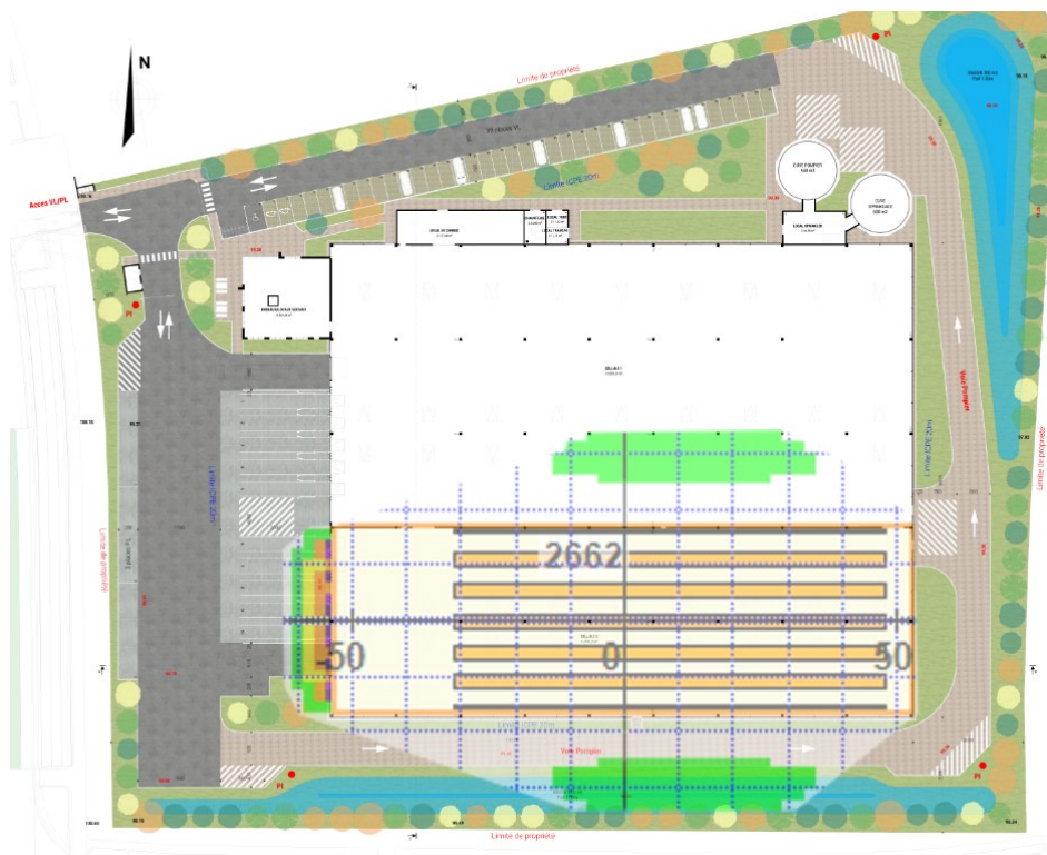
Zones d'effets thermiques : palette type 2662 - cellule 2 Stockage 8 m
