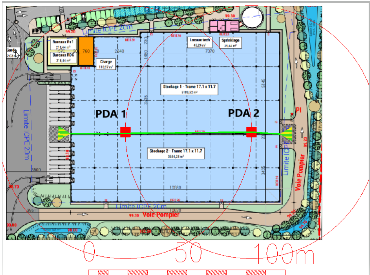
Figure 12 : Implantation des paratonnerres
