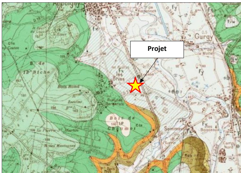
Carte géologique du secteur
