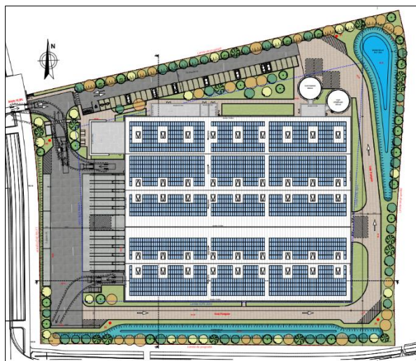
Schéma de principe de gestion des eaux pluviales
