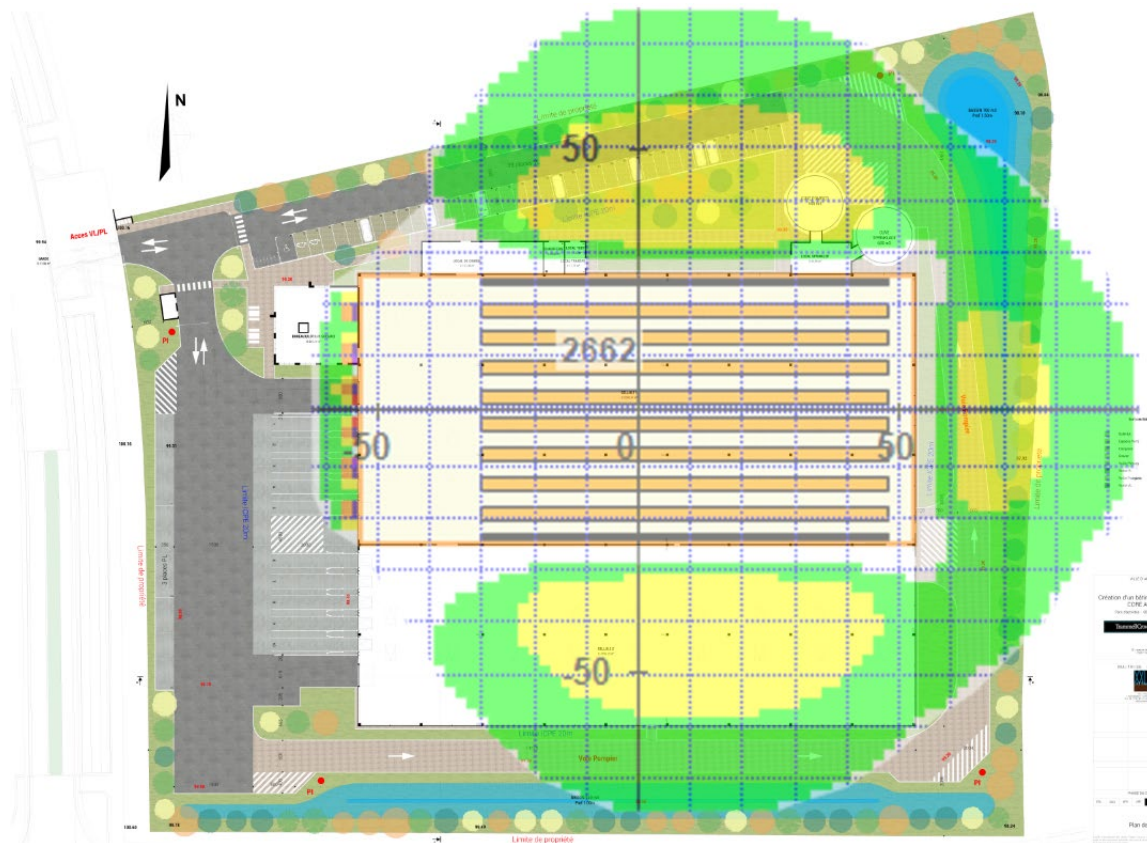
Zones d'effets thermiques : palette type 2662 - cellule 1 Stockage 11,7 m
