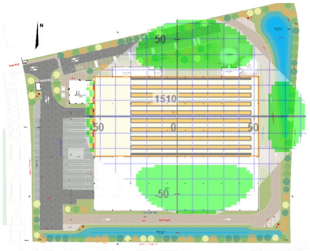
Zones d'effets thermiques : palette type 1510 - Cellule 1 Stockage 11,7 m
