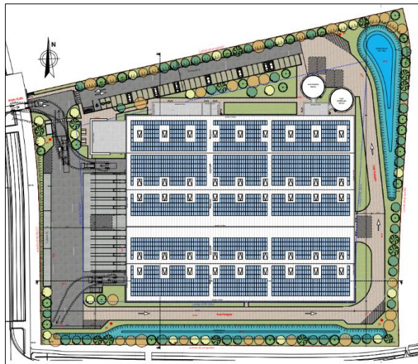
Extrait du plan d'aménagement de principe de l'opération
