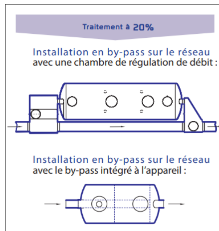
Options de configuration du déboureur séparateur d'hydrocarbures
