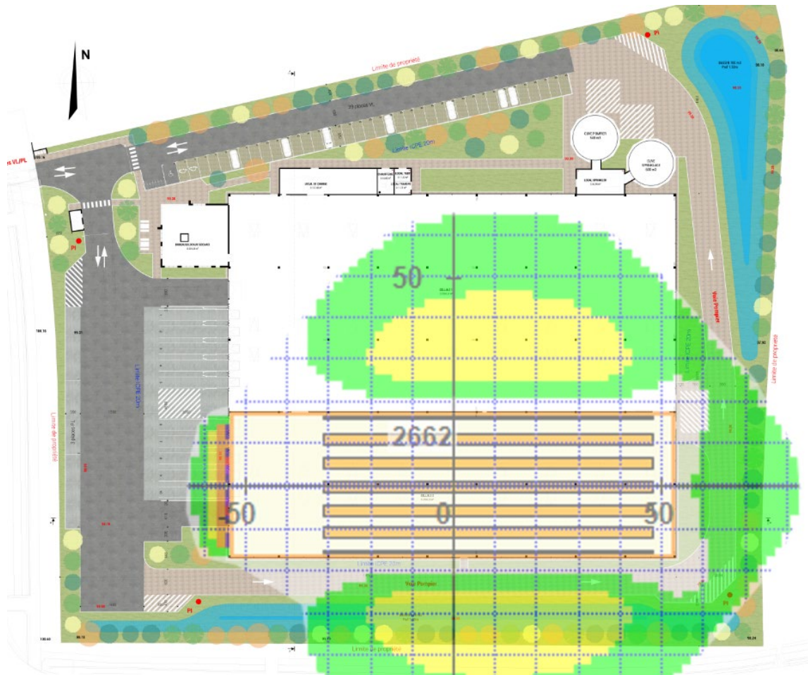
Zones d'effets thermiques : palette type 2662 - cellule 2 Stockage 11,7 m
