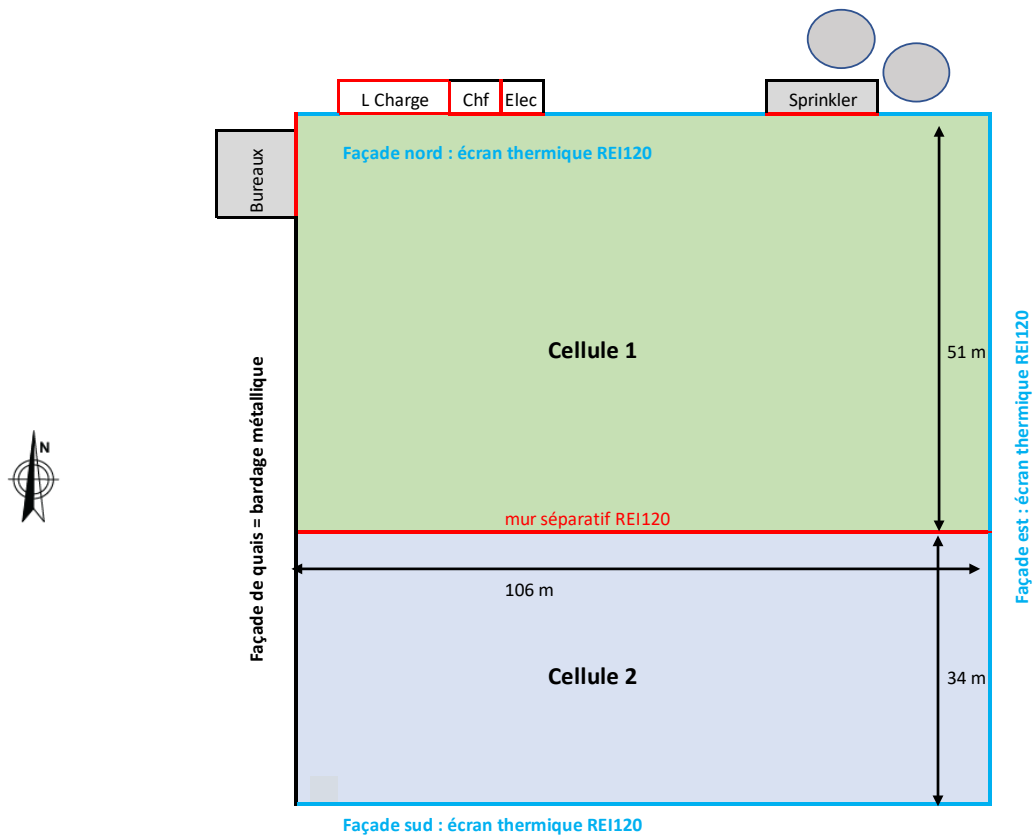
Représentation schématique du bâtiment CORE 1
